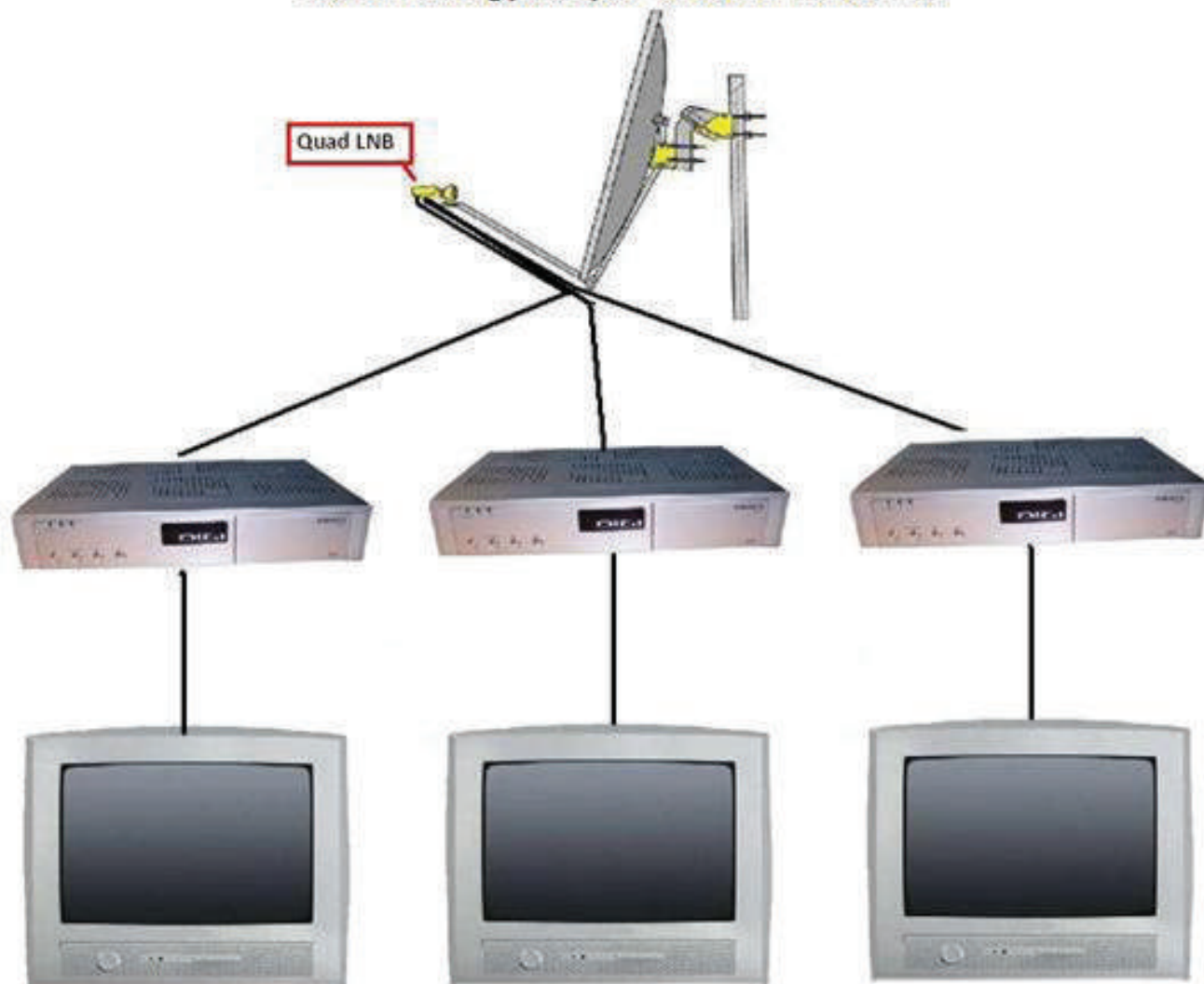
Három db egykártyás dekóder bekötése
